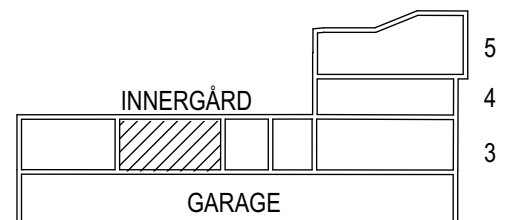
SEKTION
